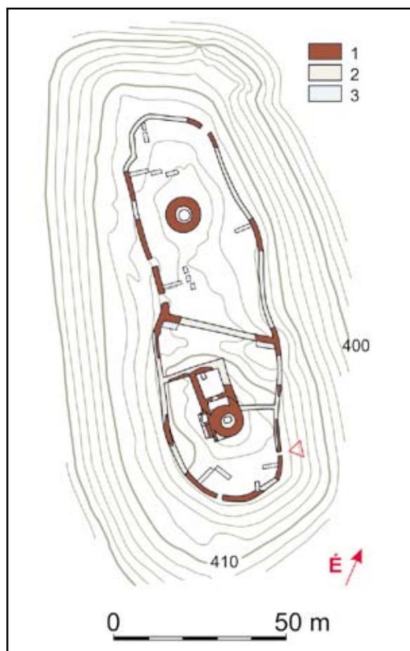
Solymos várának alaprajza az eddigi kutatások alapján (Nováki Gyula felmérésének felhasználásával készítette Szökrön Péter) 1. álló falak, 2. feltételezett falak, 3. kutatóárok
