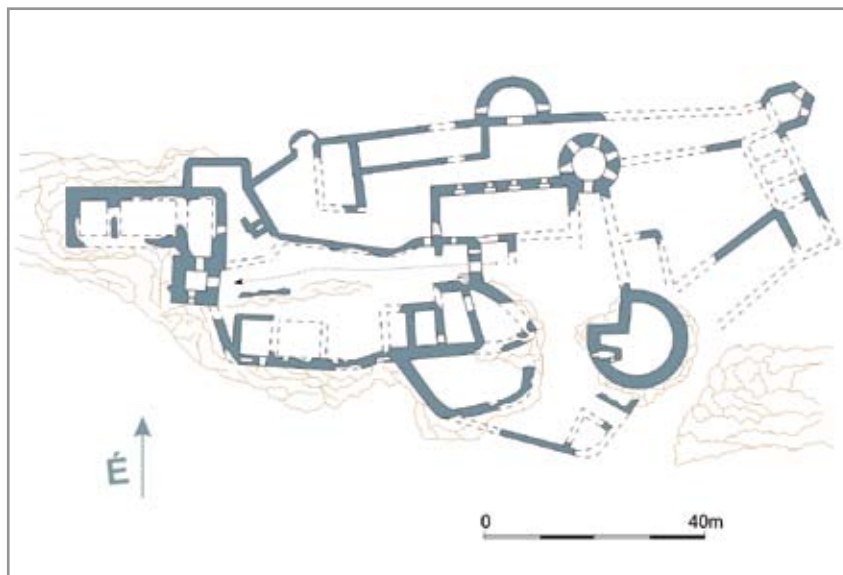
Éleskő várának alaprajza
